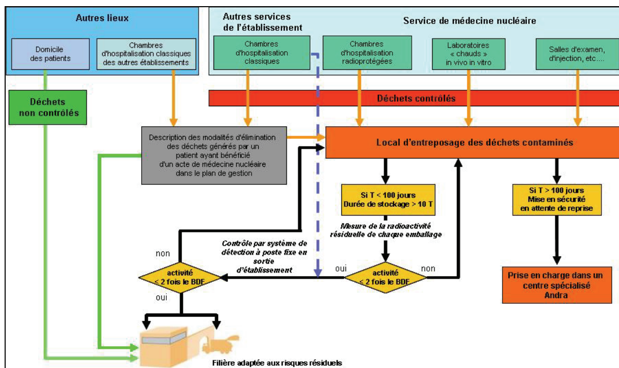
Figure 1 : la gestion des déchets contaminés par des radionucléides générés par les activités de médecine nucléaire
